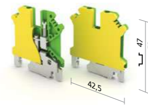
UT1-2,5PE(T)
