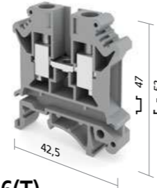
UT1-6(T)
