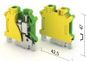
UT1-10PE(T)
